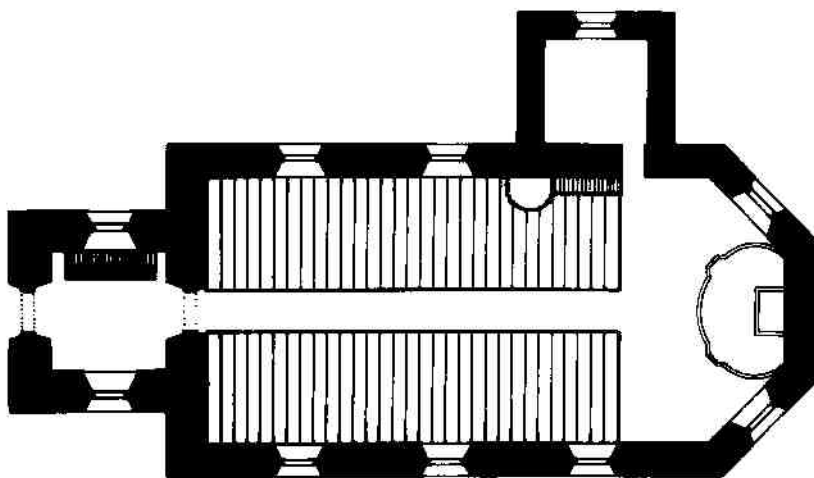
Planritning över det första kapellet. Utrymmet i kyrkan blev större, då väggarna gjordes av trä, ej av sten som å ritningen.
